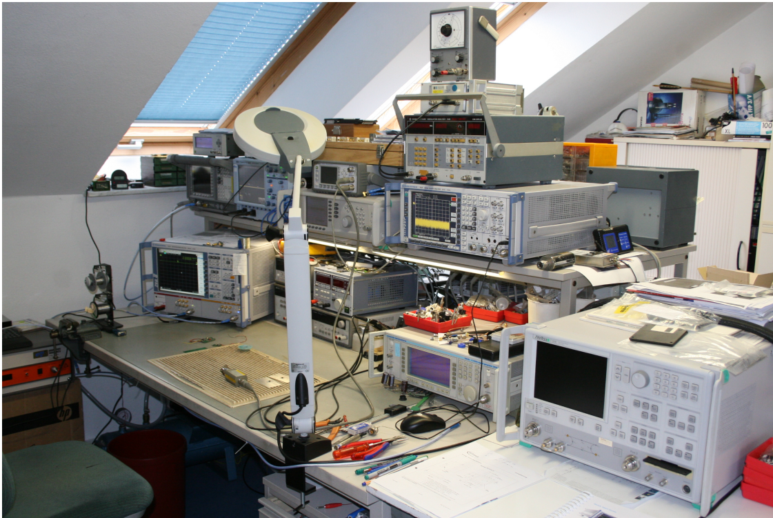
Unser Entwicklungs- und Messplatz (10Hz – 40GHz)
